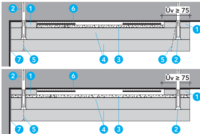
Alternativ Promat®-Reflex auf Streifen
